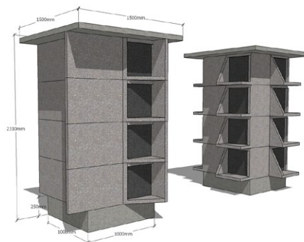
Schets model R - zuilopstelling 16 nissen
